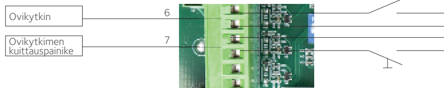
Magneettikytkin
