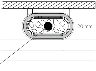
BILD 3 Skyddsavstånd till bastulaven runt bastuaggregatet på en höjd på under 900 mm.
