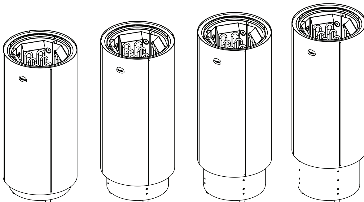
Höhe 790 mm
